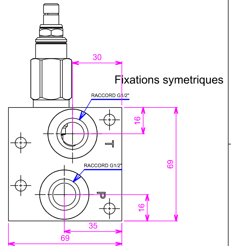
Embase NG06 sorties latérales et limiteur de pression
