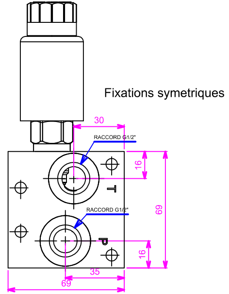
Embase NG06 sorties latérales avec distributeur de by-pass
