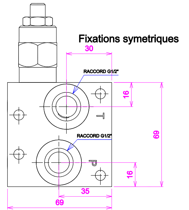
Embase NG06 sorties latérales et limiteur de pression 1DR30P20S
